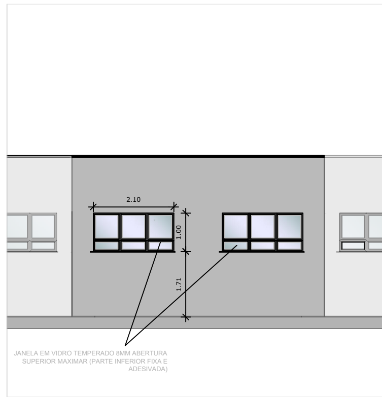
FACHADA ESC.: 1:100
