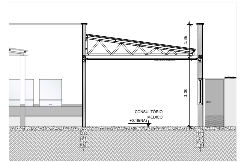
CORTE B/B ESC.: 1:100
