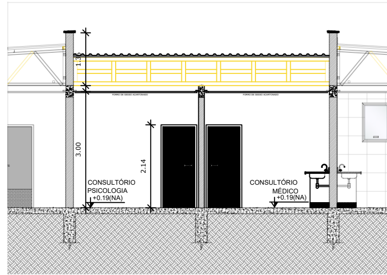
CORTE A/A ESC.: 1:100
